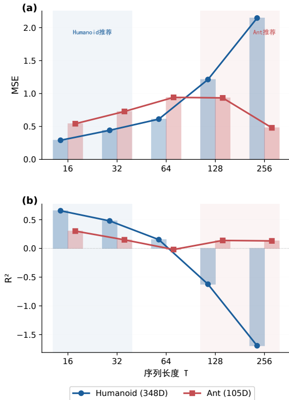
图 3 S4D-WM 在不同序列长度下的预测精度
