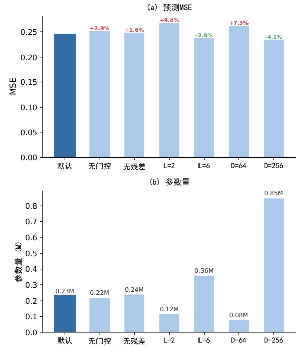
图 4 消融实验结果可视化
