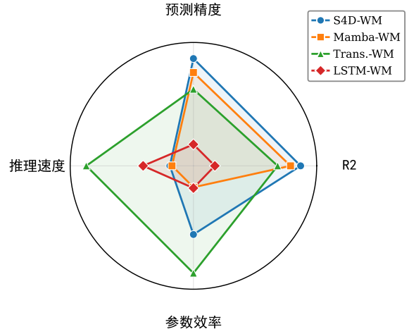
图 7 各方法多维度性能对比 (D4RL Humanoid)
