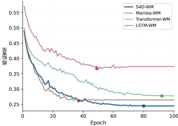
图 5 各模型 D4RL Humanoid 训练曲线
