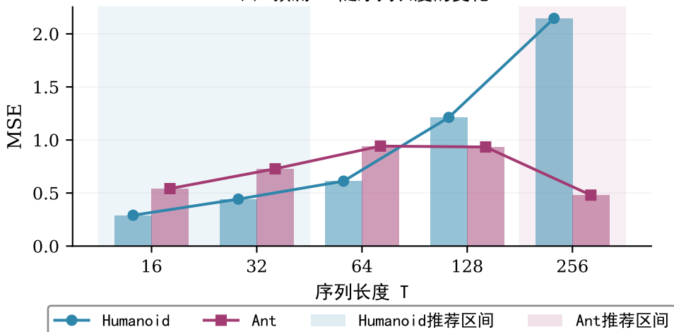
(a) 预测MSE随序列长度的变化
