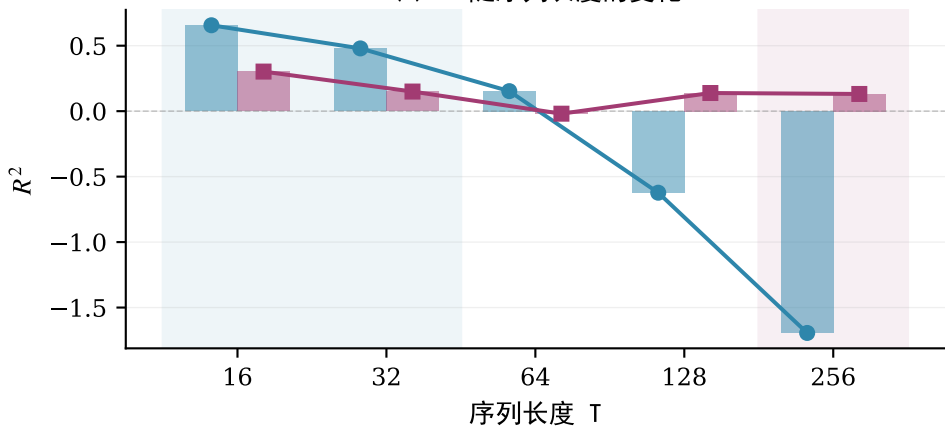
(b) R^2 随序列长度的变化
