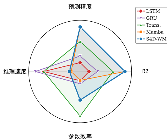
图 3 各方法多维度性能对比 (Humanoid)
