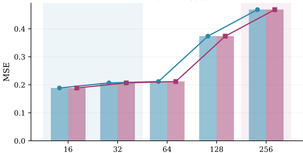
(a) 预测MSE随序列长度的变化
