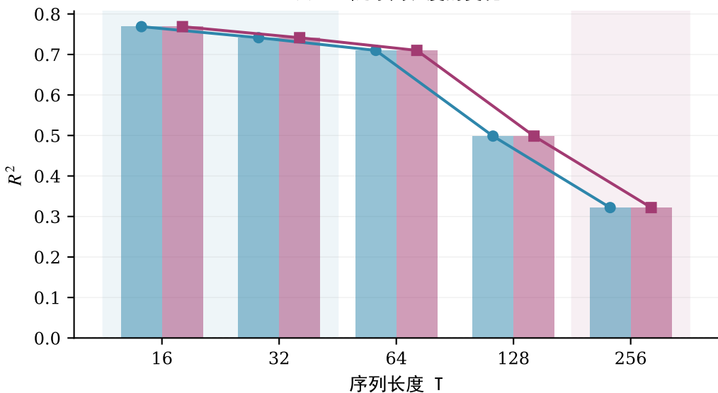
(b) R^2 随序列长度的变化
