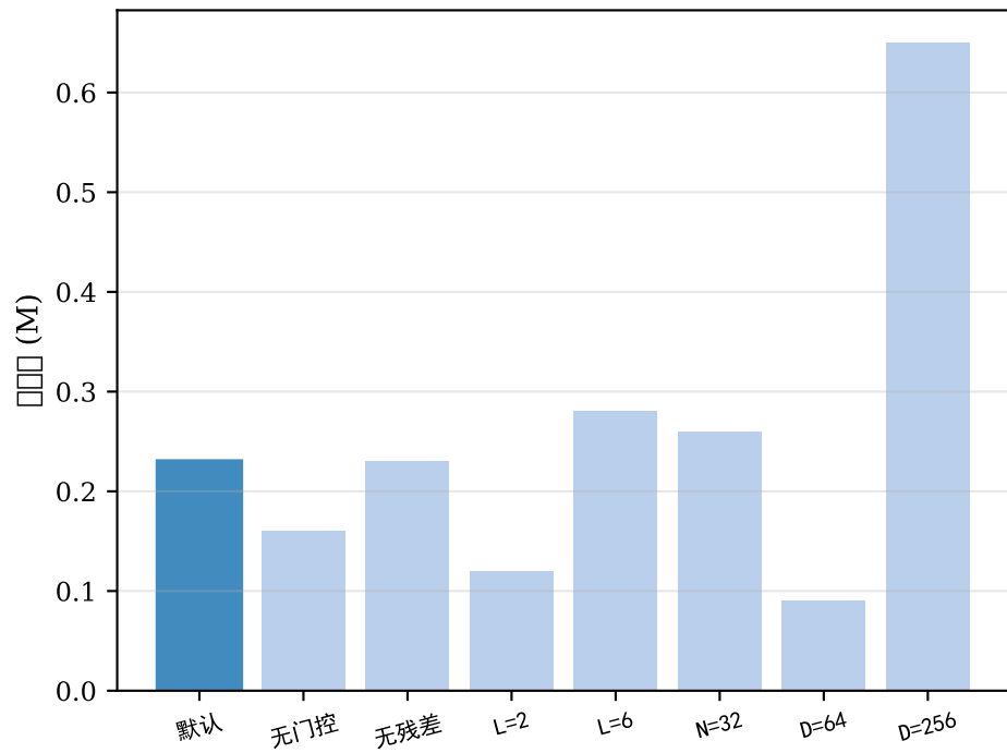
(b) 参数量
