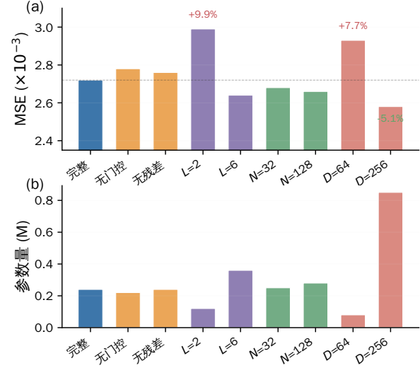
图4 消融实验结果可视化
