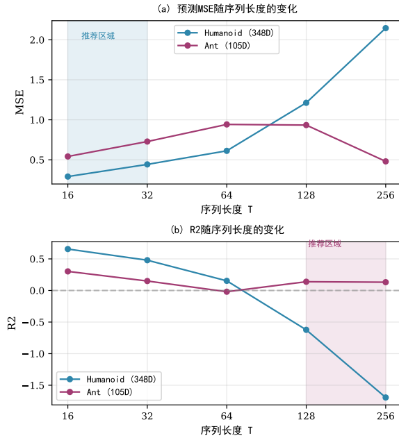
图 3 S4D-WM 在不同序列长度下的预测精度
