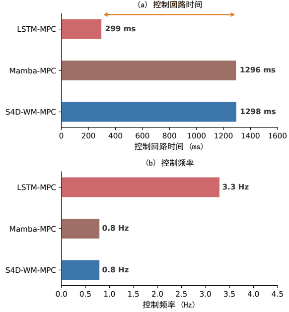
图5 MPC 控制性能对比
