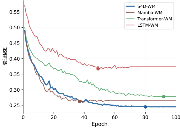
图4 各模型 D4RL Humanoid 训练曲线
