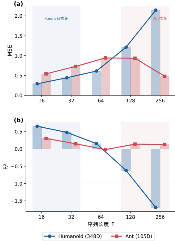
图2 S4D-WM 在不同序列长度下的预测精度
