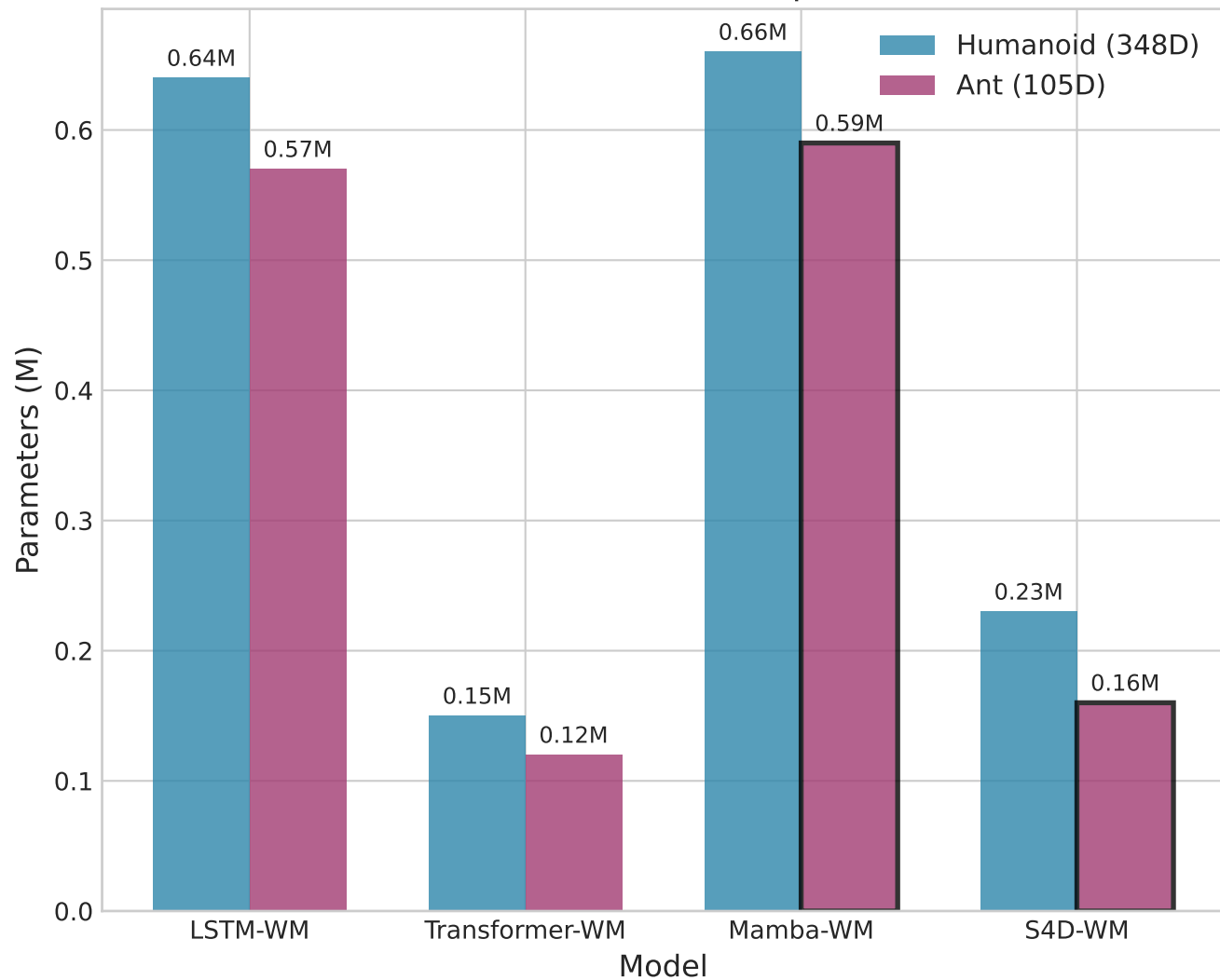
Parameter Count Comparison
