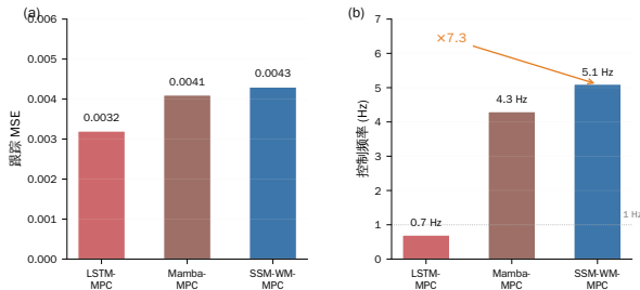
图 6 MPC 控制性能对比
