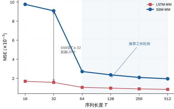
图3 预测 MSE 随序列长度变化趋势
