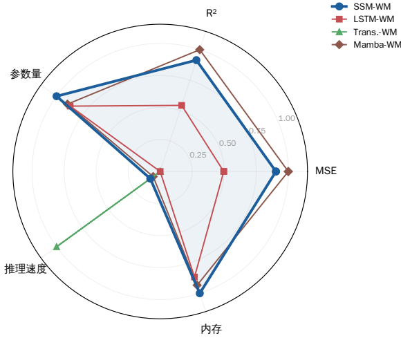
图 7 各方法多维度性能雷达图对比
