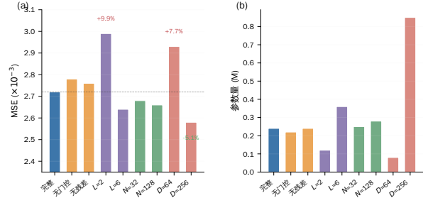
图4 消融实验结果可视化
