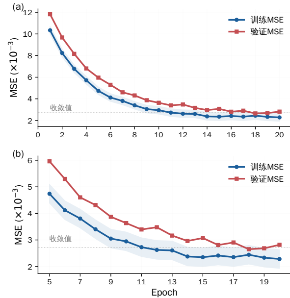
图 4 S4D-WM 训练曲线 (阴影区域表示训练 MSE 的 \pm 标准差)
