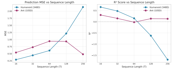
图 2 S4D-WM 在不同序列长度下的预测精度
