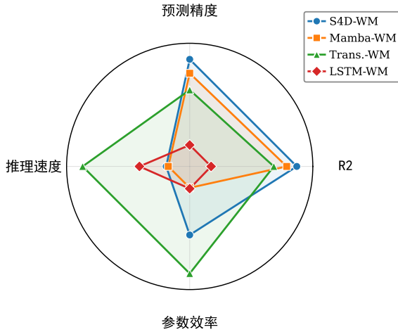
图 6 各方法多维度性能对比 (D4RL Humanoid)
