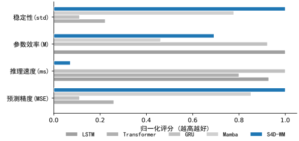
图 7 各方法多维度性能对比 (D4RL Humanoid)
