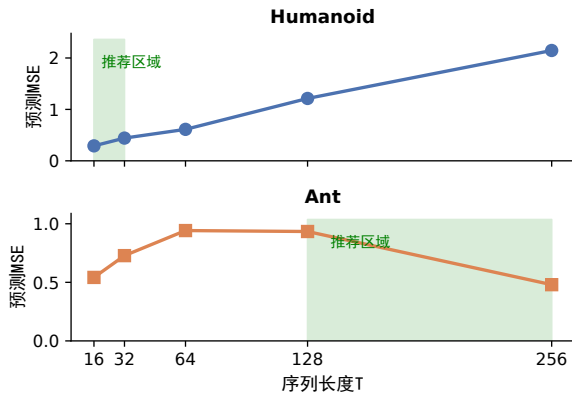
图 3 S4D-WM 在不同序列长度下的预测精度
