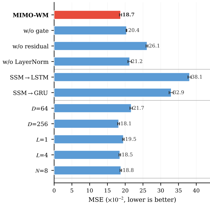
(a) MSE
