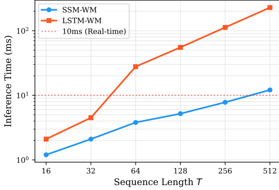
图 4 推理时间随序列长度变化趋势
