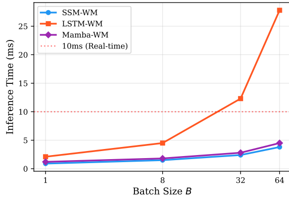
图 3 不同批次大小下的推理时间对比
