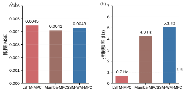
图 5 MPC 控制性能对比
