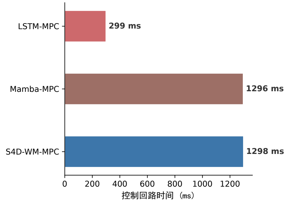
(a) 控制回路时间
