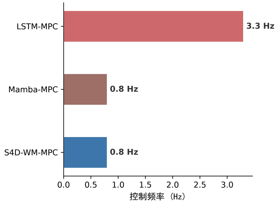
(b) 控制频率
