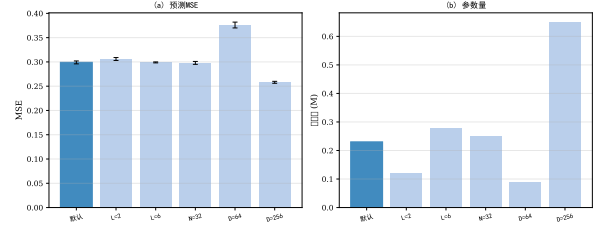
图5 消融实验结果可视化
