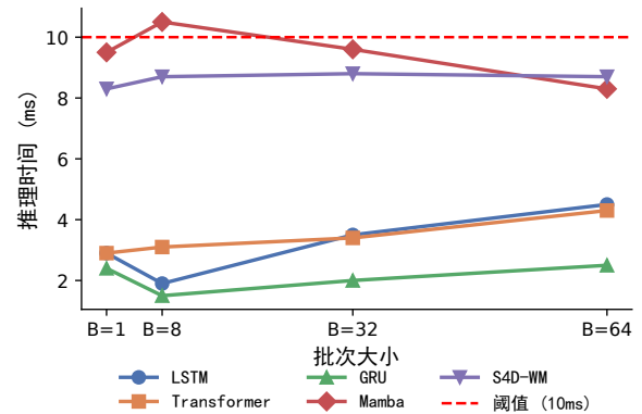
图 2 不同批次大小下的推理时间对比
