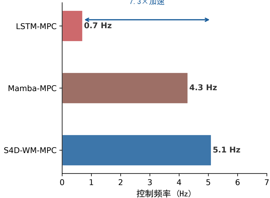
(b) 控制频率 7.3×加速
