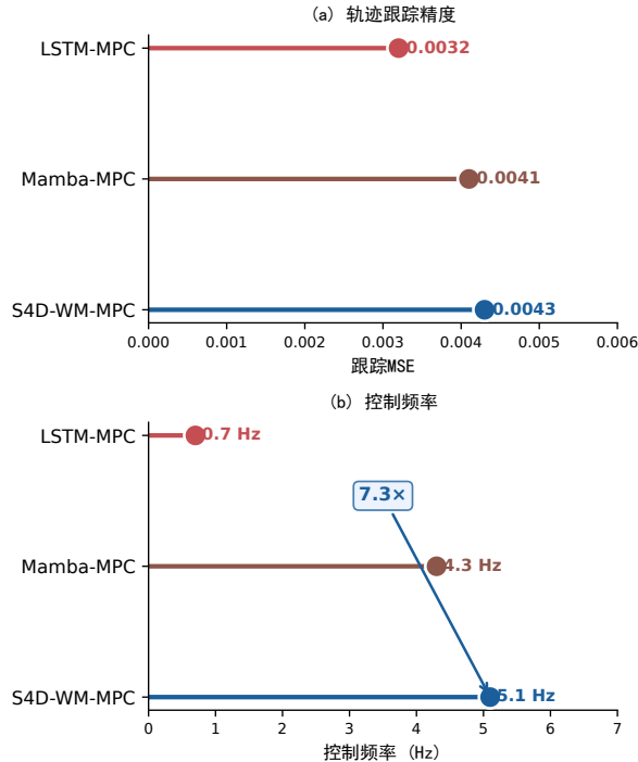
图 5 MPC 控制性能对比
