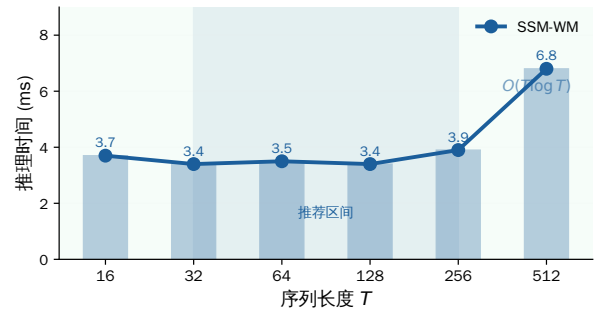
图 2 推理时间随序列长度变化趋势
