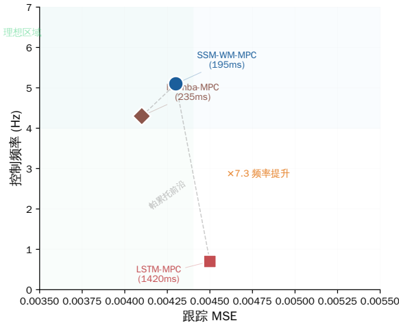
图 5 MPC 控制性能对比
