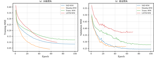
图 4 各模型 D4RL Humanoid 训练曲线
