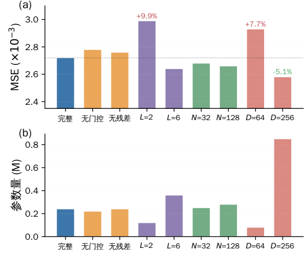
图 5 消融实验结果可视化 (D4RL Humanoid)
