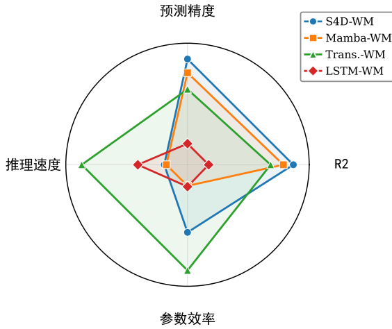
图6 各方法多维度性能对比 (D4RL Humanoid)
