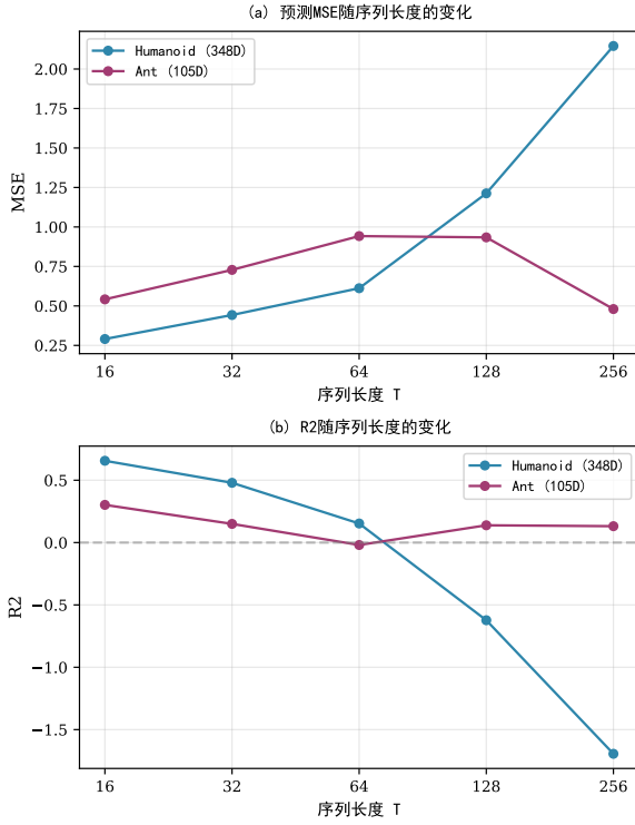
图2 S4D-WM在不同序列长度下的预测精度
