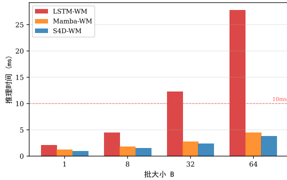
图 1 不同批次大小下的推理时间对比
