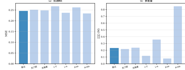
图3 消融实验结果可视化
