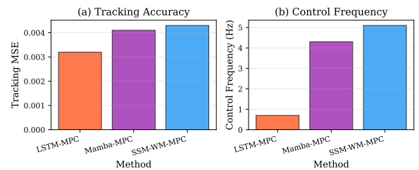
图 7 MPC 控制性能对比
