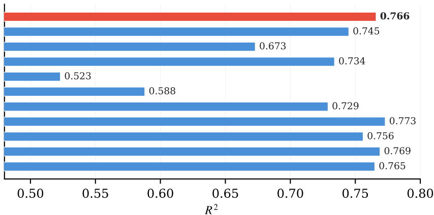
(c) Parameters
