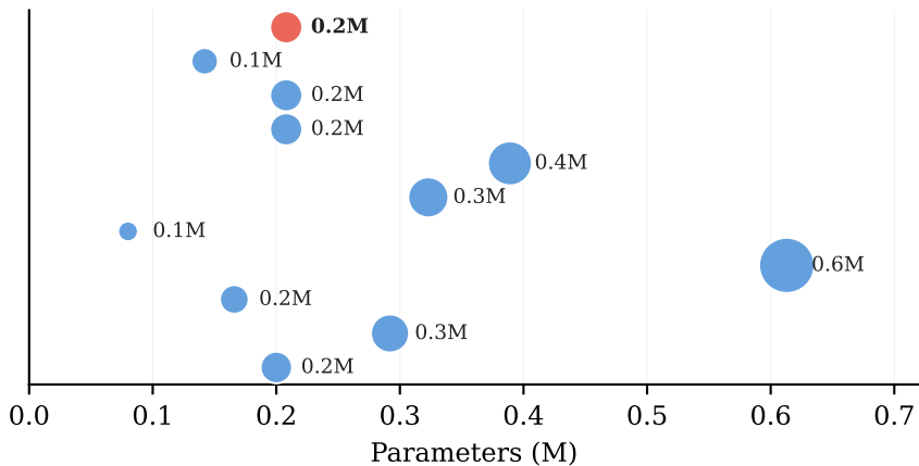
(c) Parameters
