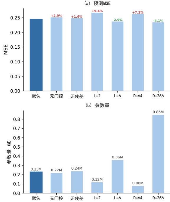
图 5 消融实验结果可视化
