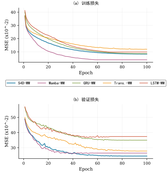
图 6 各模型 D4RL Humanoid 训练曲线
