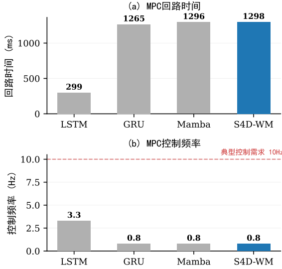
图 7 MPC 控制性能对比
