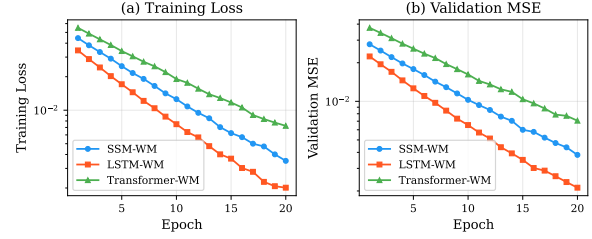
图 2 SSM-WM 训练曲线 (合成数据集)
