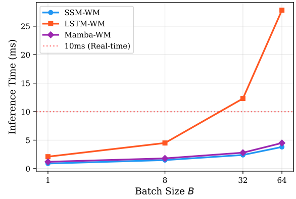
图 3 不同批次大小下的推理时间对比
