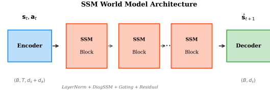
图 1 SSM 世界模型架构
