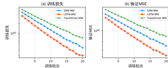
图 5 SSM-WM 训练曲线 (合成数据集)
