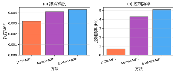
图 6 MPC 控制性能对比
