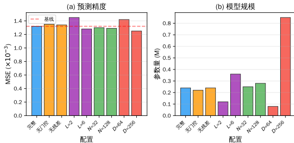
图 4 消融实验结果可视化 study results visualization
