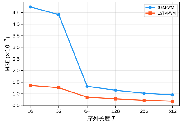
图 3 预测 MSE 随序列长度变化趋势
