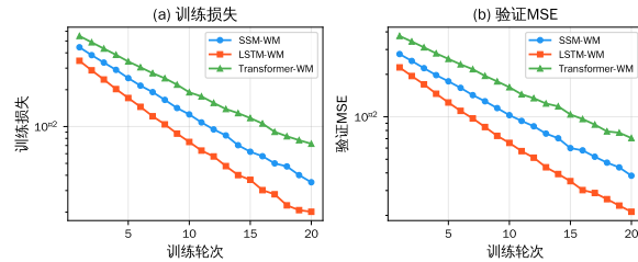
图 5 SSM-WM 训练曲线 (合成数据集) curves of SSM-WM (synthetic dataset)
