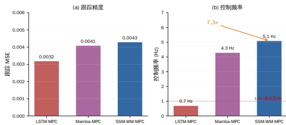
图 6 MPC 控制性能对比
