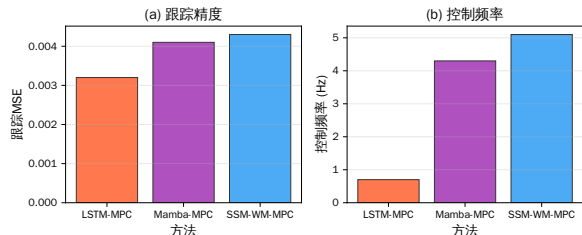
图 6 MPC 控制性能对比
