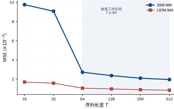
图 3 预测 MSE 随序列长度变化趋势
