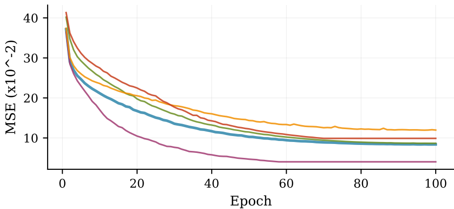
(a) 训练损失
