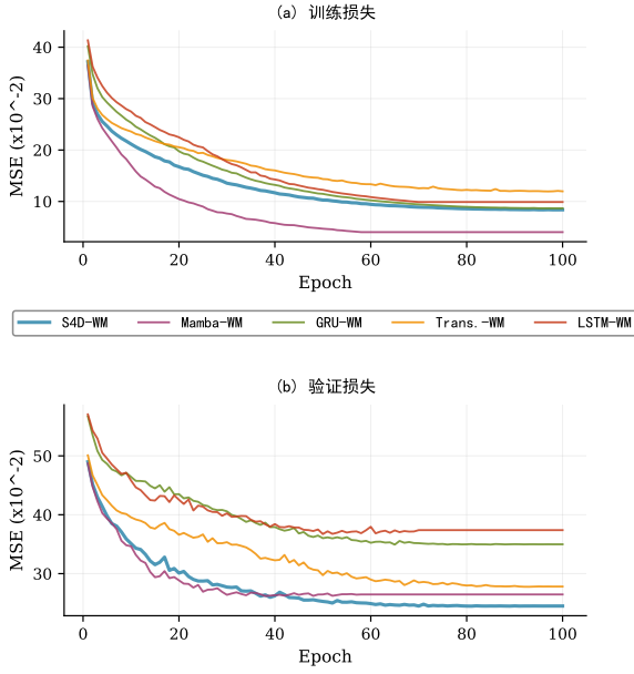
图 6 各模型 D4RL Humanoid 训练曲线
