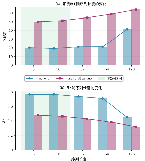
图 4 序列长度敏感性分析
