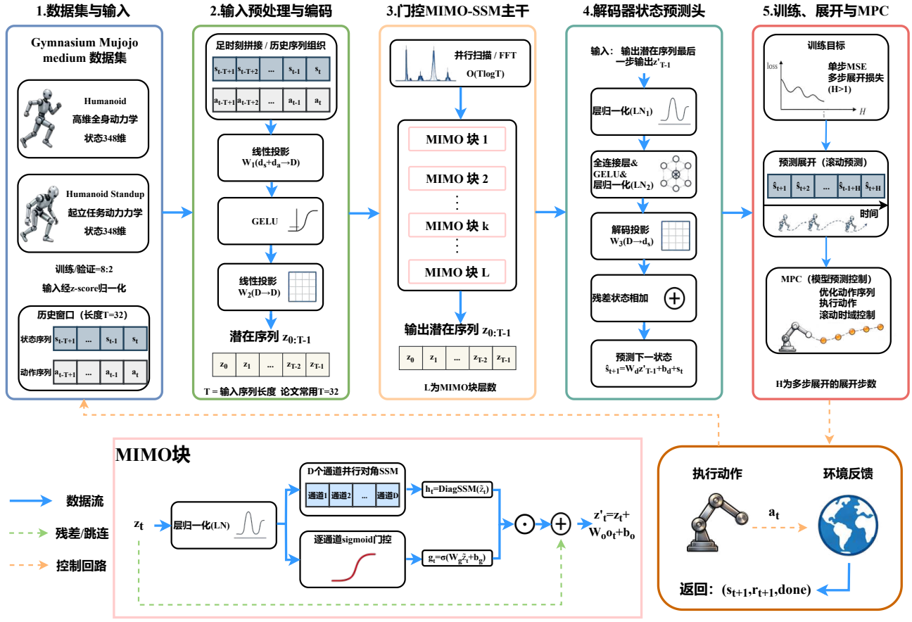
图 1 MIMO-WM 整体架构
