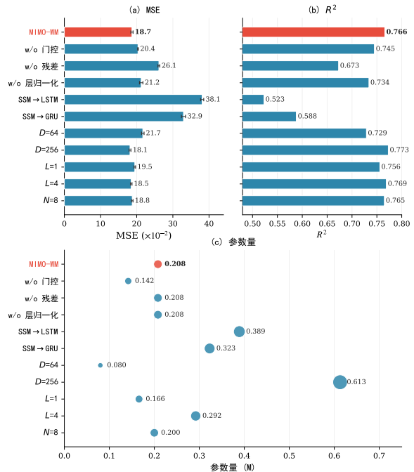
图 3 消融实验结果可视化
