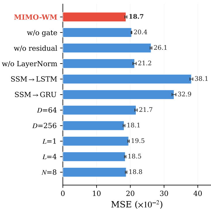
(a) MSE
