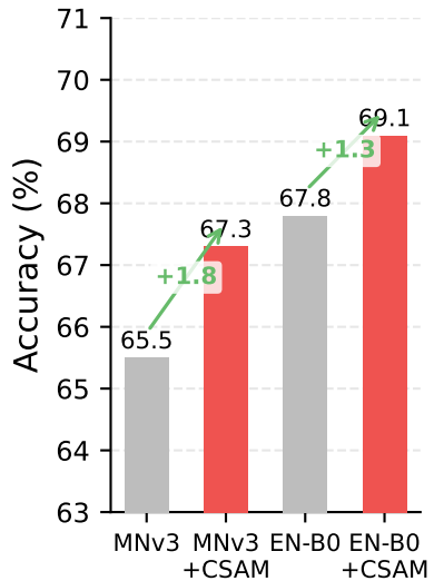
(d) CSAM Effect
