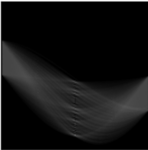
Parameter space
