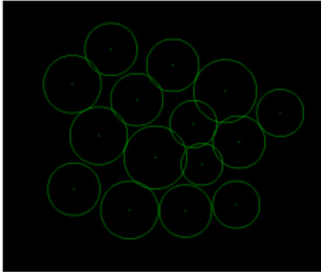
scikit-image Circles
