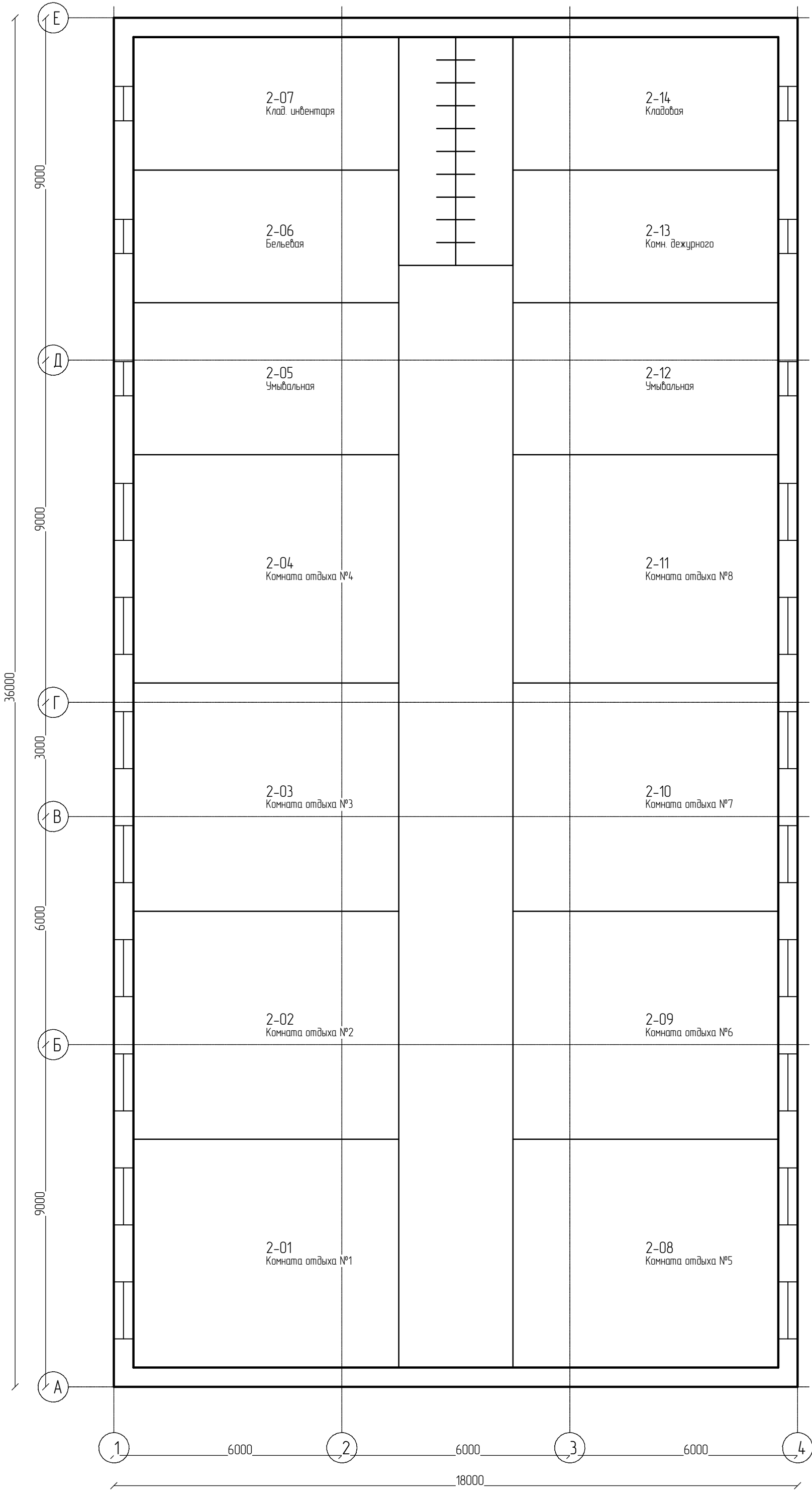
План 2-го этажа М 1:100
