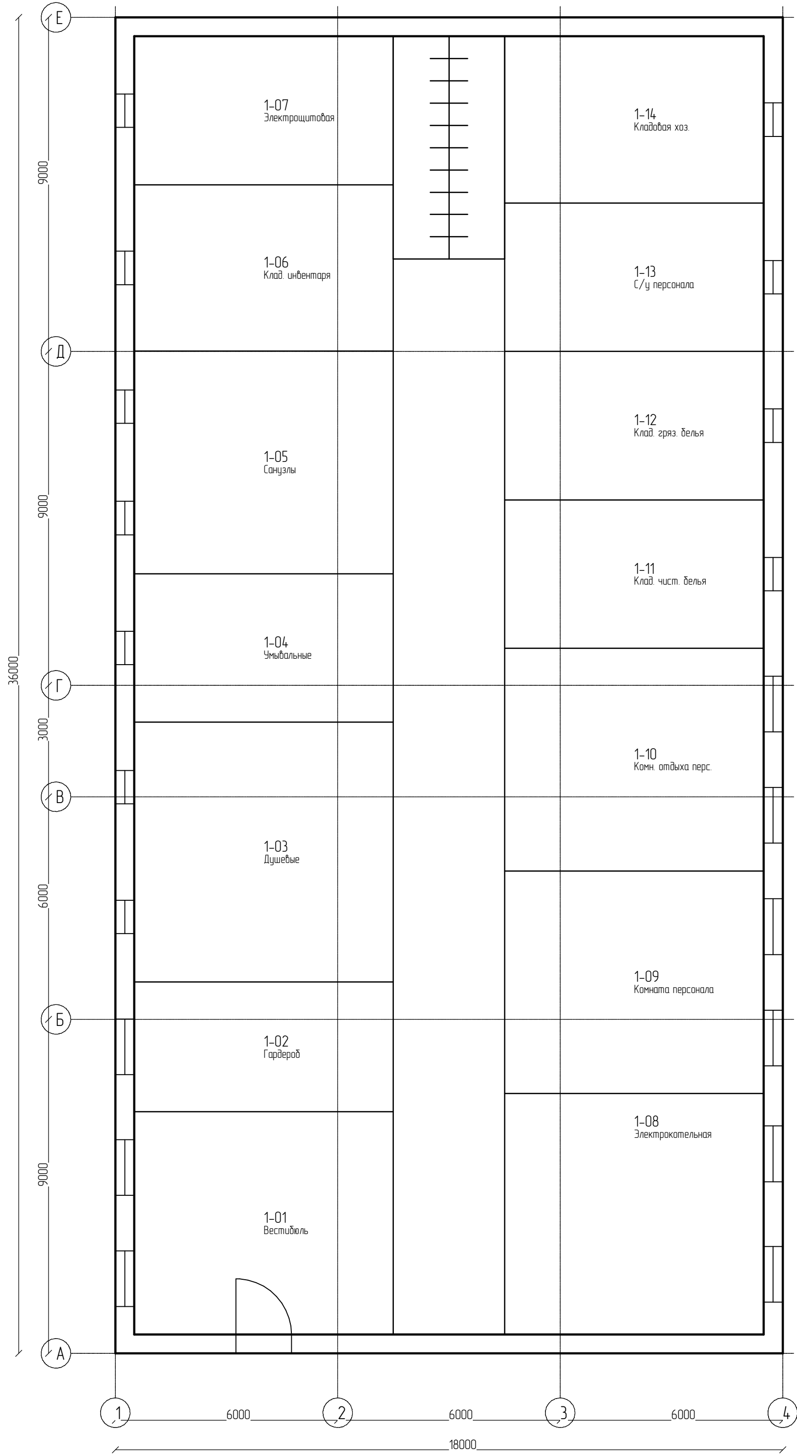
План 1-го этажа М 1:100
