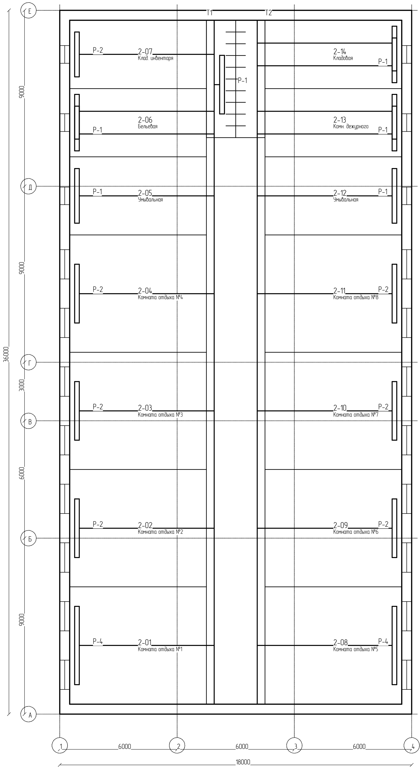
План 2-го этажа. Система отопления М 1:100
