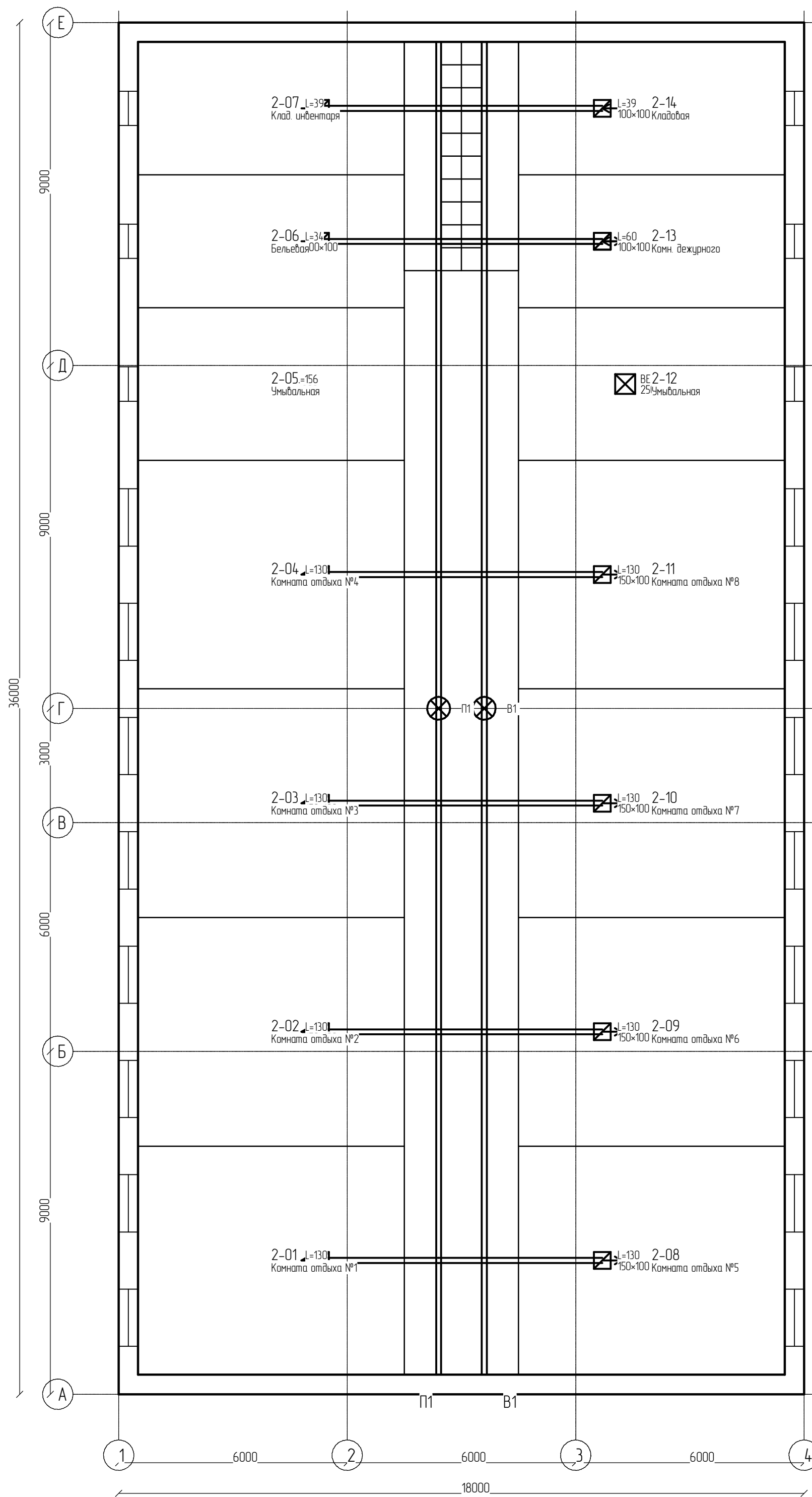
План 2-го этажа. Система вентиляции М 1:100
