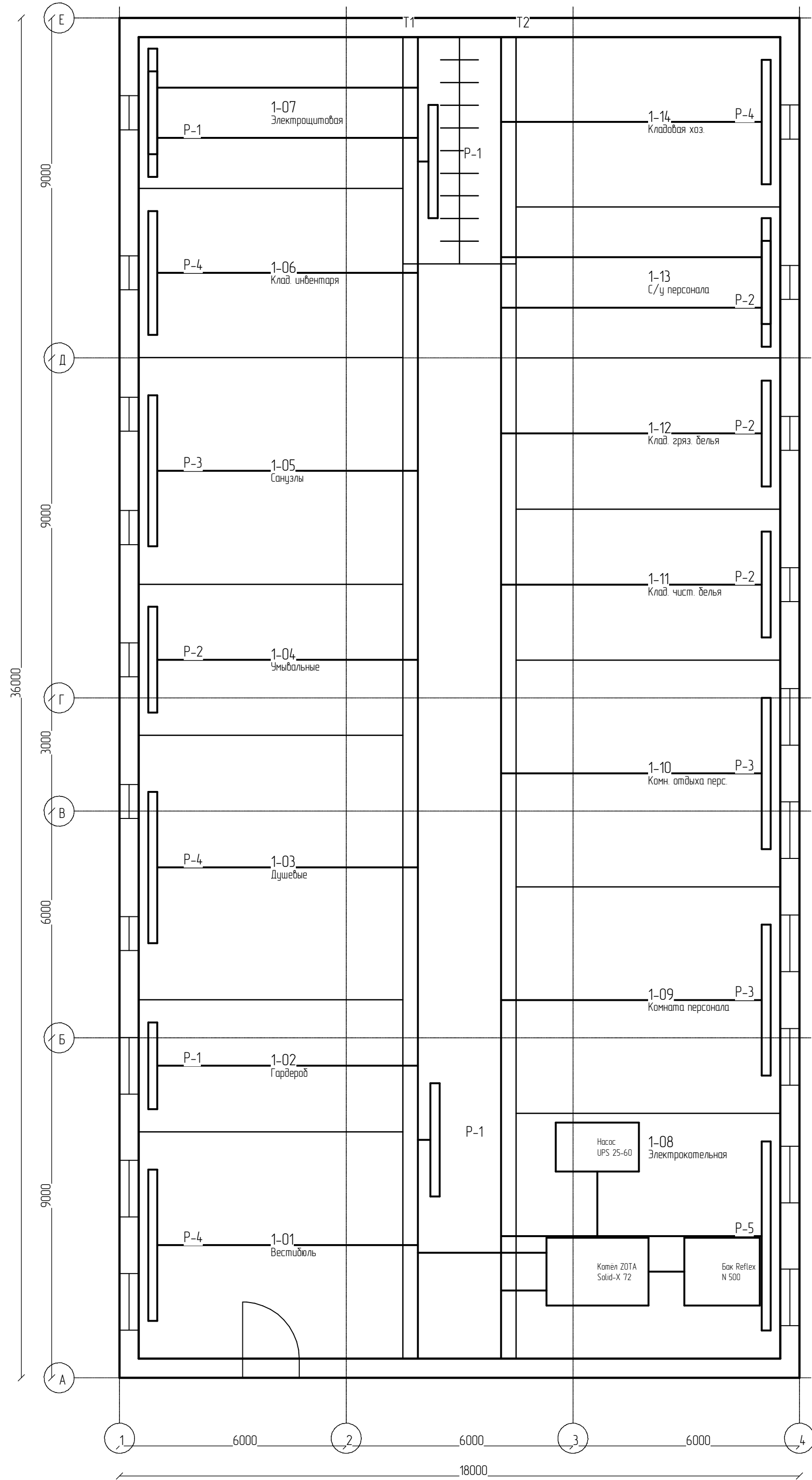
План 1-го этажа. Система отопления М 1:100
