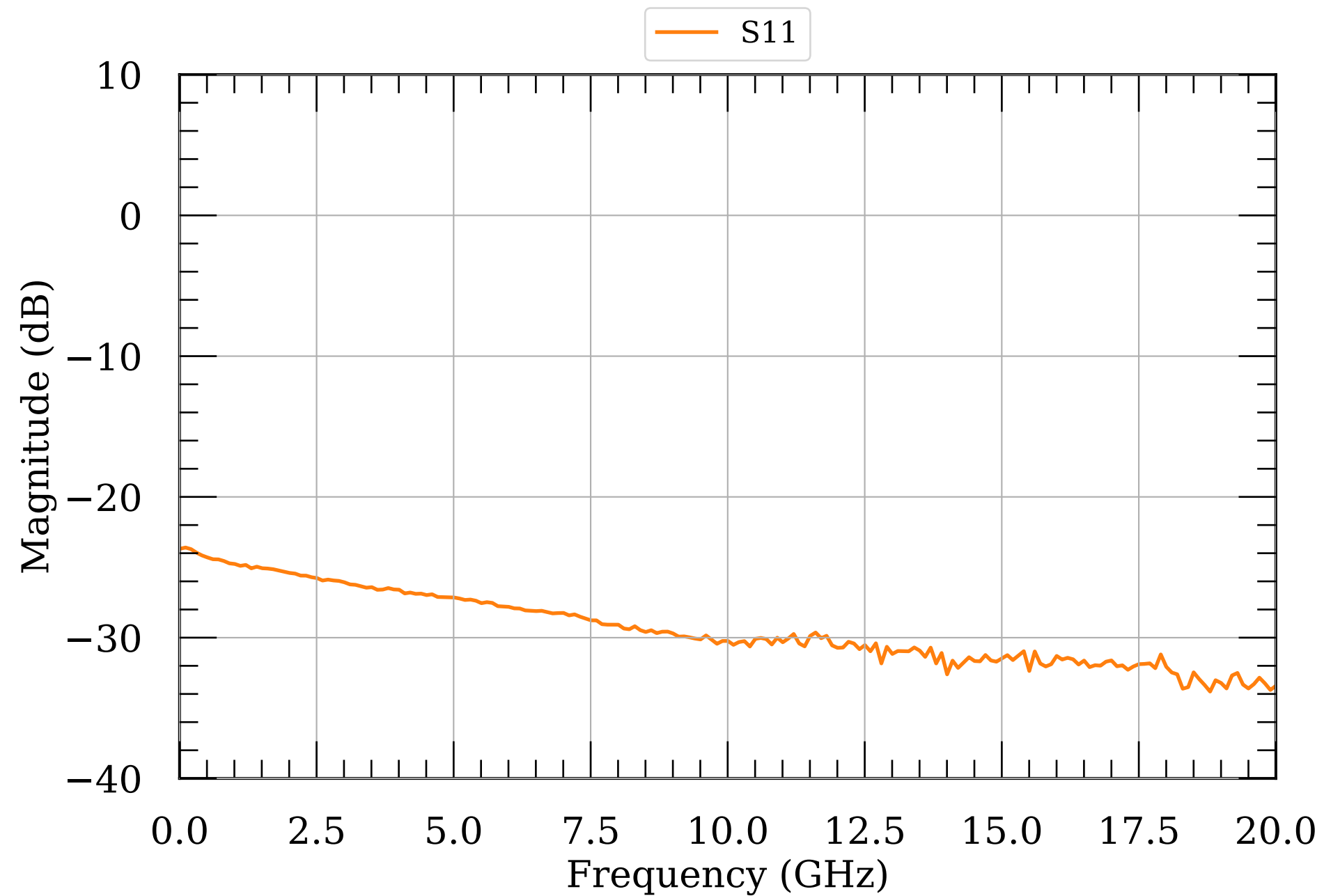
LNA S-params 21.0
