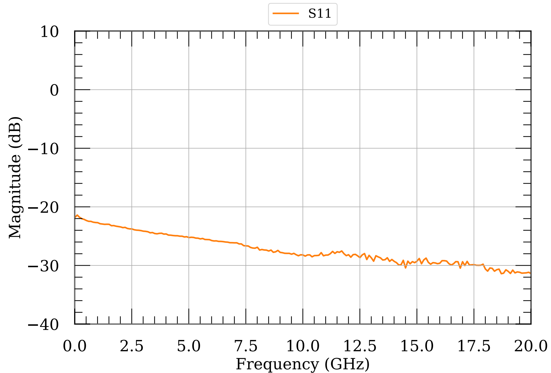
LNA S-params 25.0
