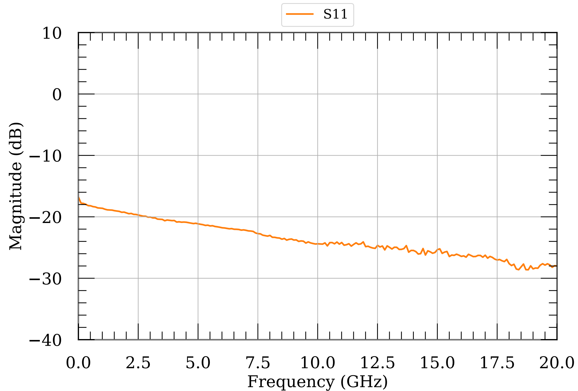
LNA S-params 30.5
