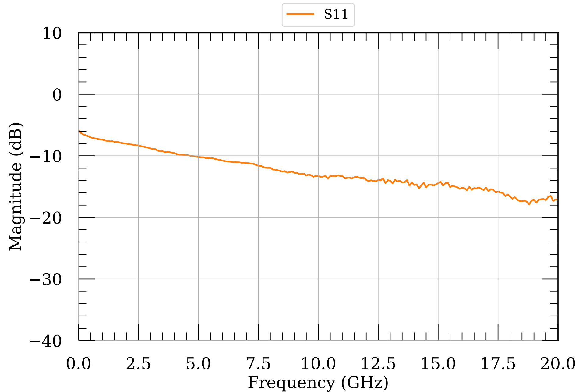
LNA S-params 4.5
