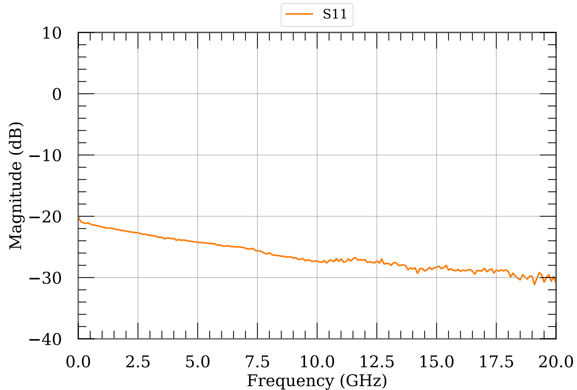
LNA S-params 9.0
