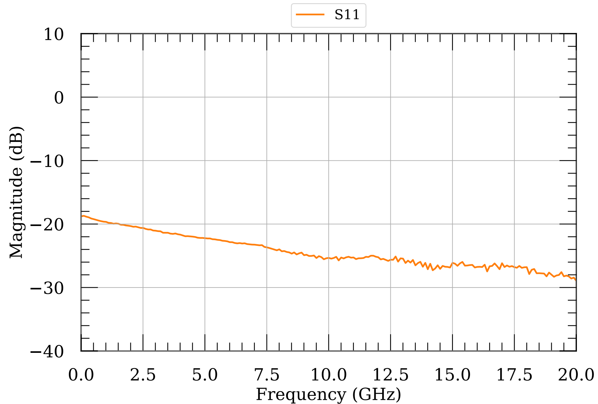
LNA S-params 1.5
