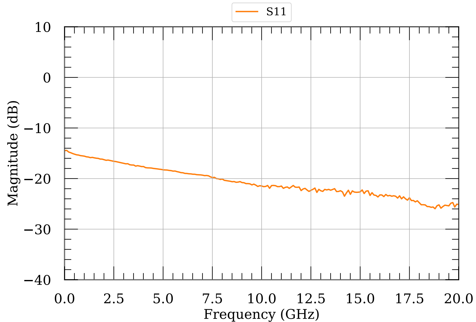
LNA S-params 6.0
